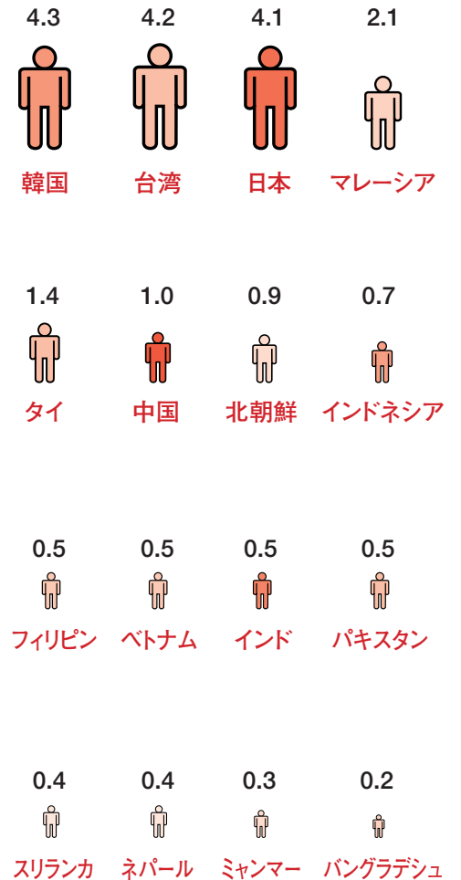
一人あたりのエネルギー消費量 (石油換算トン/人)
